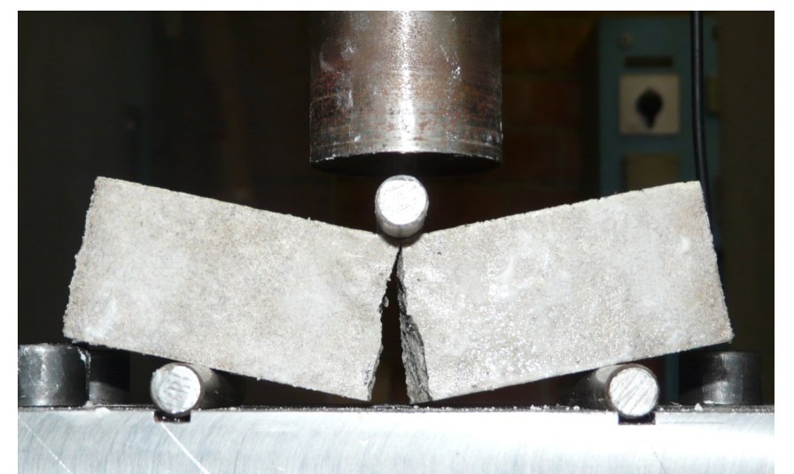
Test de résistance à la flexion
