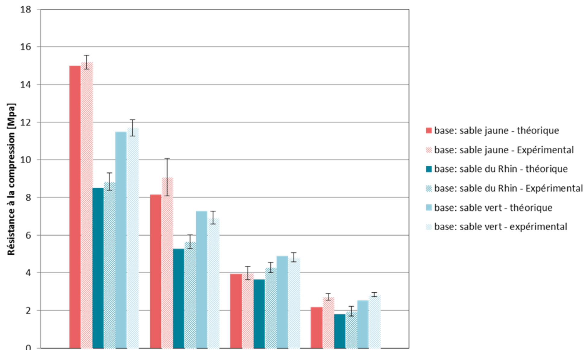
Test de résistance à la compression
