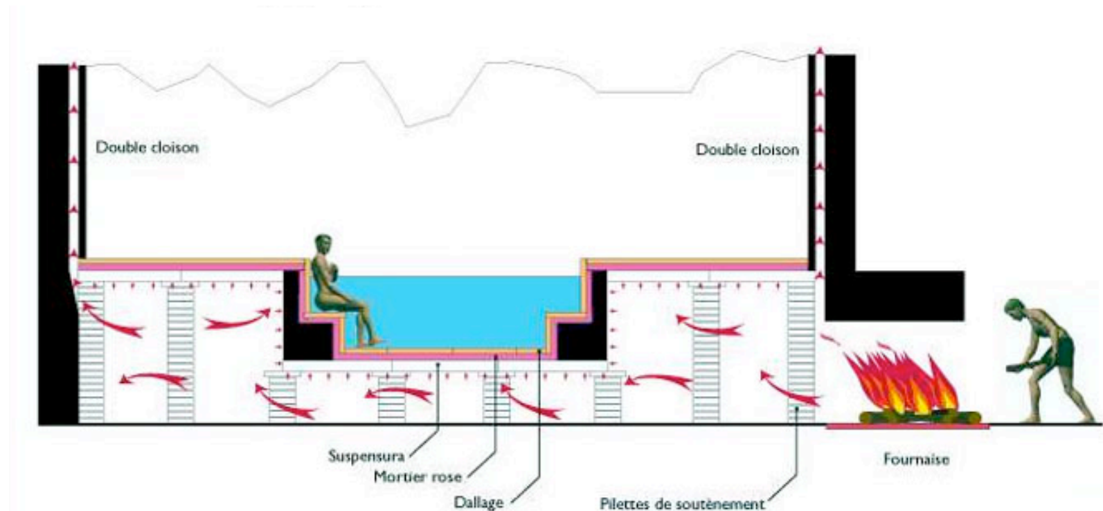
Schéma de chauffage par Hypocauste dans la Rome Antique.
