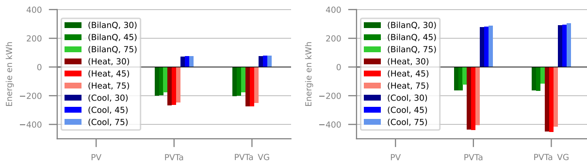
Figure 8 : Différence en kWh du bilan énergétique (BilanQ), de la chaleur utile pour le chauffage (Heat) et le refroidissement (Cool) entre la situation 1996 et celle de 1970 (à gauche) et entre 2014 et 1970 (à droite) pour une orientation sud-est et un débit auxiliaire de 150 \text{ m}^3/\text{h}
